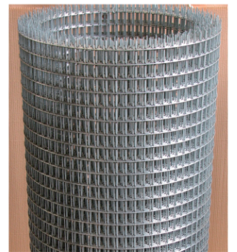
2.0φ x 30 x 20
