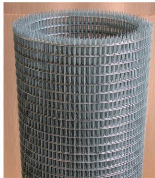
2.0φ x 30 x 15
