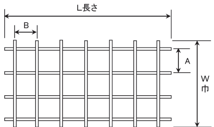
2.0φ x 30 x 15
